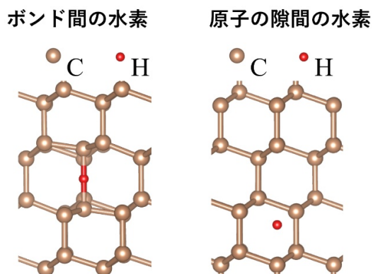
ダイヤモンド内部の水素の配置
