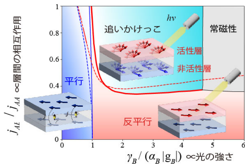
図 2 本研究で提案した手法を二層の磁性金属を接合した系に適用したときの相図。光を当てていないときに平行であった二層の磁性が、光を当てることで反平行になったり、追いかっこする状態になったりする。
