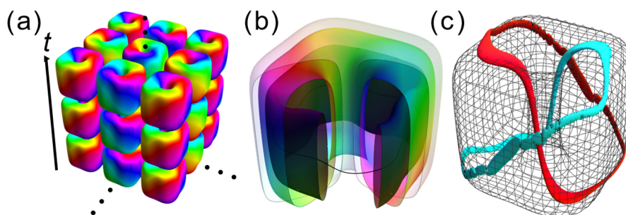
図3 (a) 計算された3次元時空ホプフィオン結晶。(b) 単位構造および(c) その横偏光(赤色)と縦偏光(水色)の分布。
